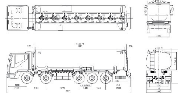
32KL BLS 외관 사면도
