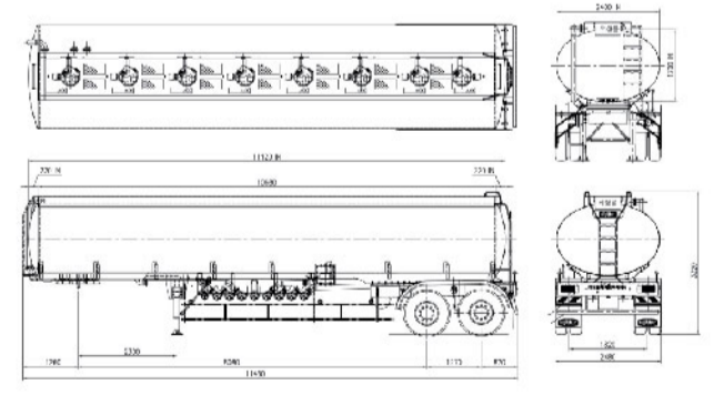
32KL BLS 외관 사면도
